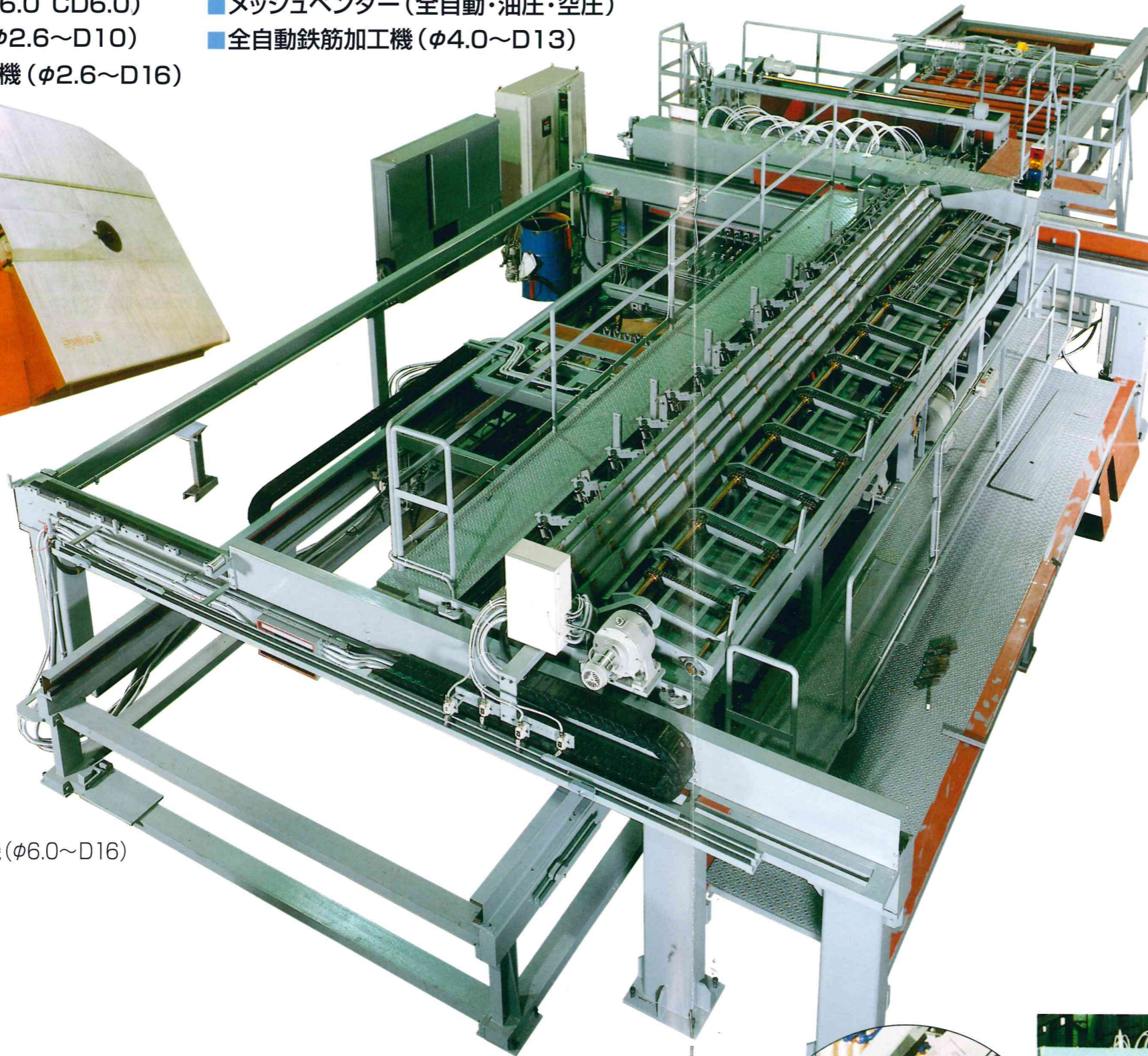
MEP全自動鉄筋加工機
