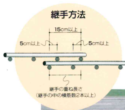
■防獣用金網(イノシシ・シカ等)
